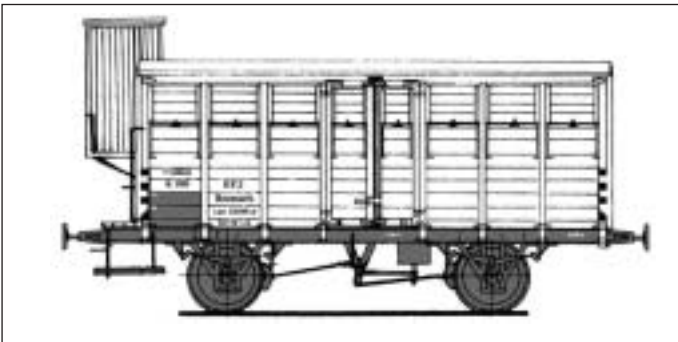
HFJ 108 Gedäckt Güterwagen mit Bremserhaus
