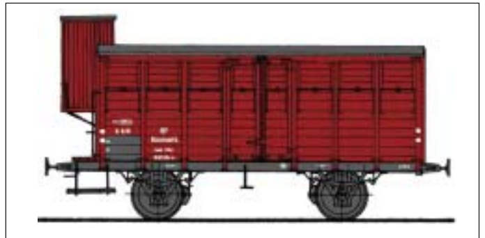
HP Q119 Gedäckt Güterwagen mit Bremserhaus
